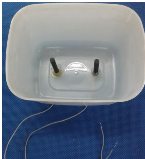
Figura 3: Recipiente reutilizado demonstrando a colocação dos eletrodos de grafite e os condutores elétricos utilizados para conexão com a fonte de alimentação da corrente contínua.
