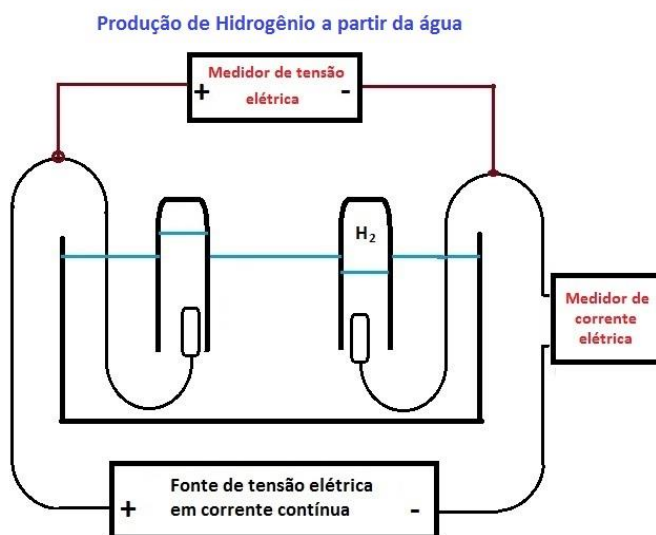
Figura 1: Representação do conjunto de materiais utilizados e como foram interligados para obter o hidrogênio e medir as grandezas elétricas envolvidas. No experimento realizado em sala de aula, os medidores elétricos não são necessários.
