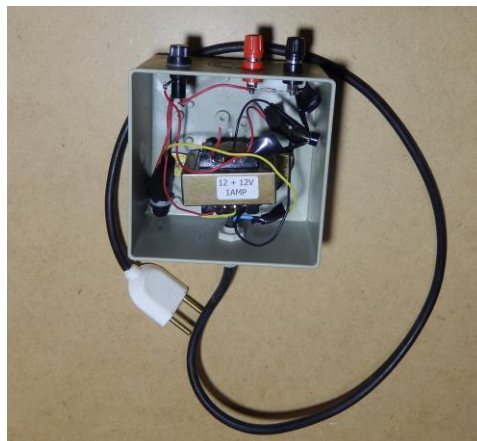
Figura 4: Interior da caixa onde foi montado a fonte de alimentação com tensão contínua.
